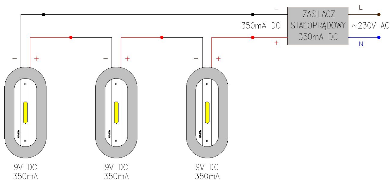
Schemat podłączenia kilku lamp za pomocą zasilacza APC-12-350
