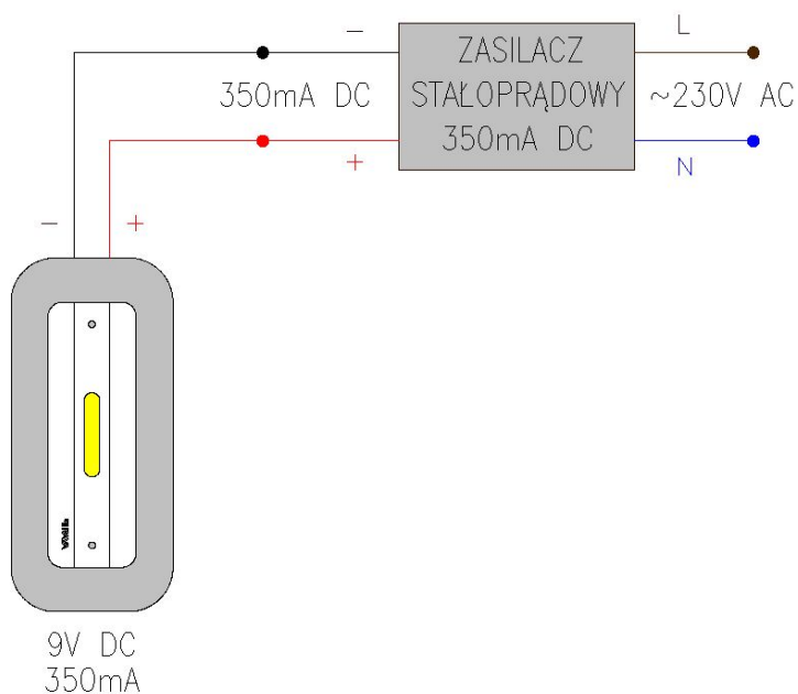
Schemat podłączenia jednej lampy za pomocą zasilacza APC-12-350
