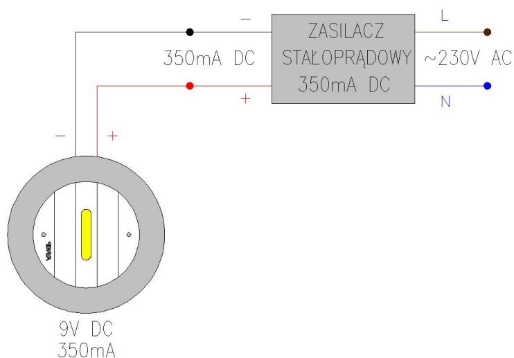
Schemat podłączenia jednej lampy za pomocą zasilacza APC-12-350
