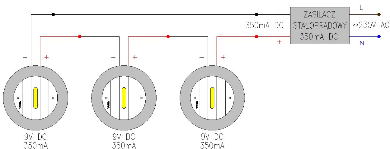
Schemat podłączenia kilku lamp za pomocą zasilacza APC-12-350
